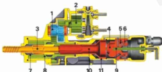
Poprečni presjek glavnih rezervnih dijelova / Top hammer drifter
